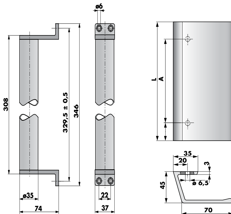
Poignée de porte "S"
