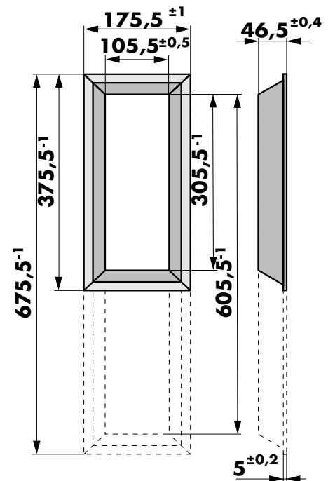
Oculus 100 x 300 (600) mm
