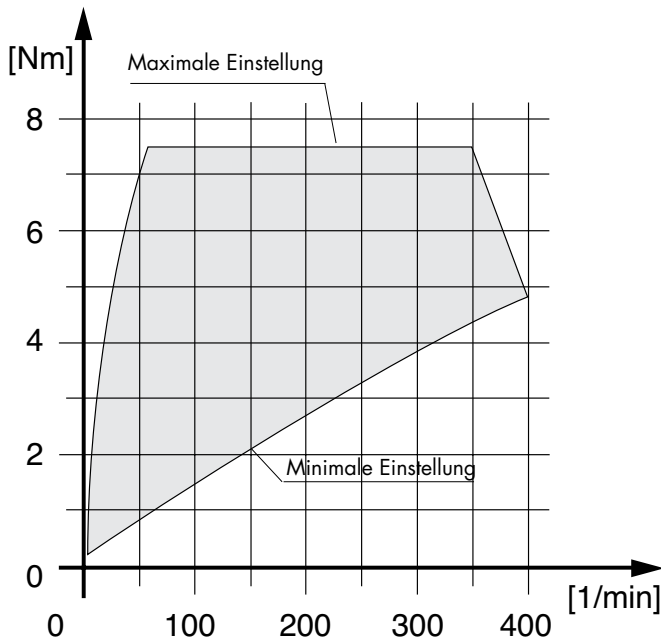
Radialdämpfer 240 / 241
