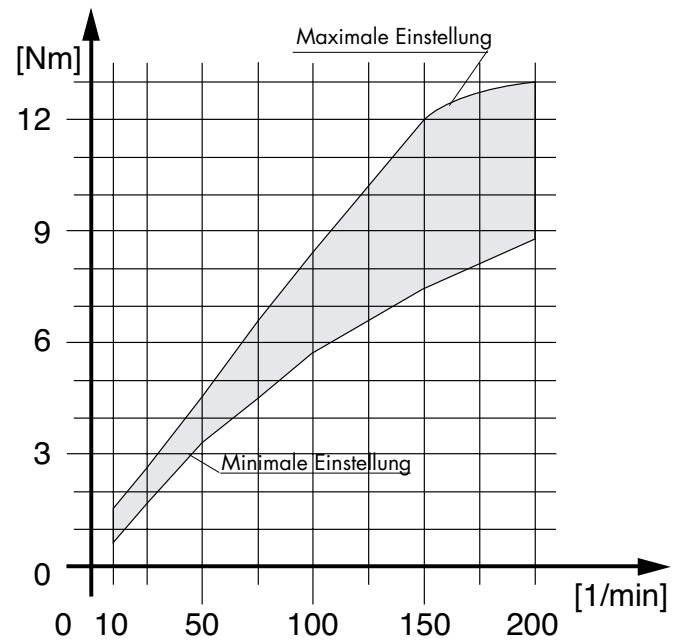
Radialdämpfer 241024 / 241030 ("Doppel-Radialdämpfer")
